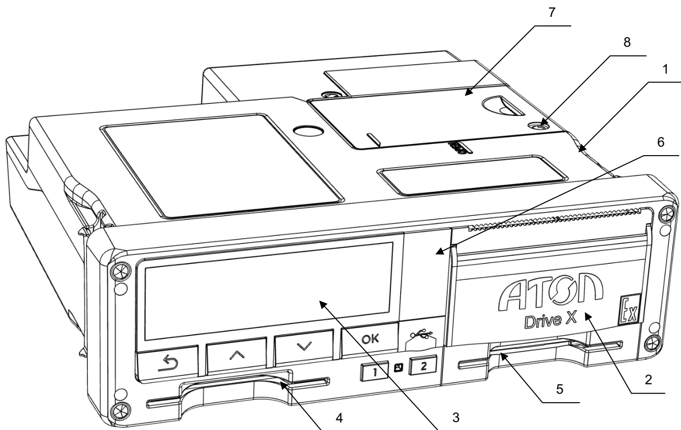
Рисунок 2. Внешний вид тахографа
