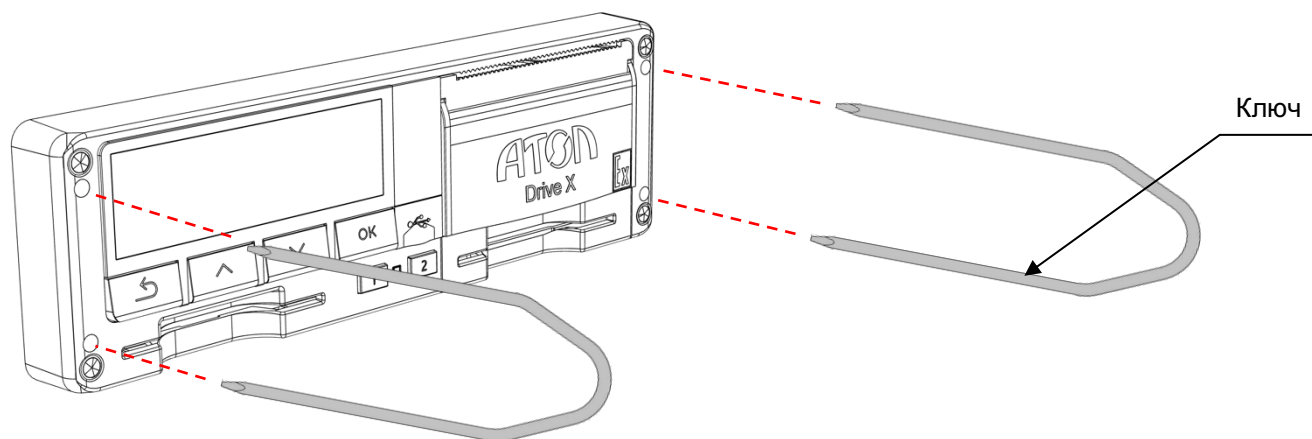
Рисунок 1. Извлечение тахографа
