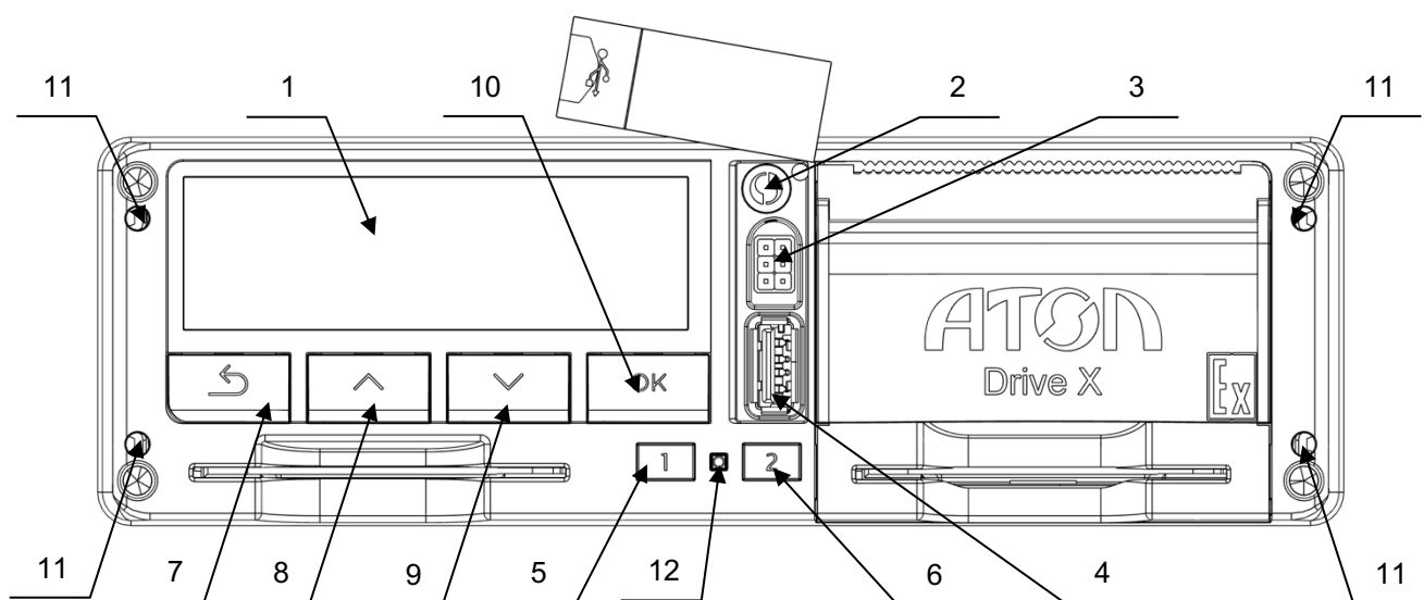
Рисунок 3. Вид спереди
