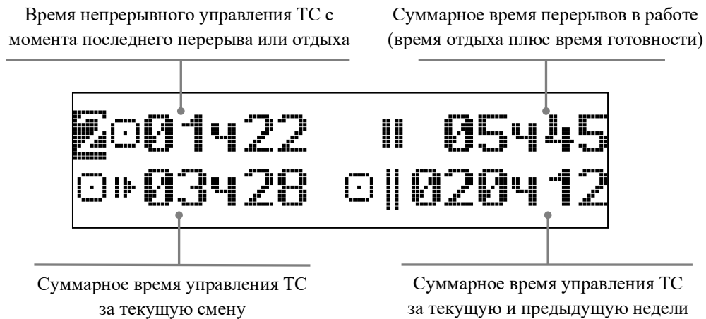
Рисунок 11. Экран «Водитель 2»
