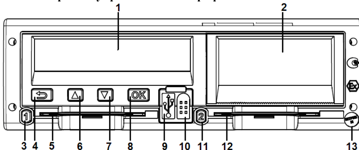
Рисунок 2 – Внешний вид передней панели тахографа SM100.42.00.00.15
